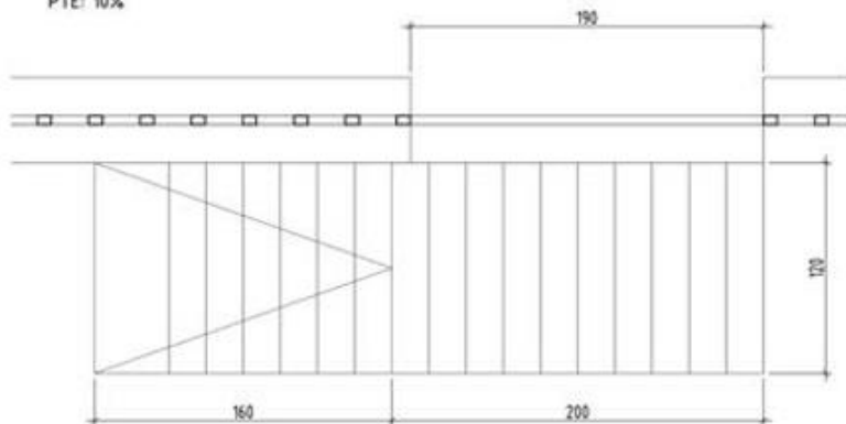
Planta
