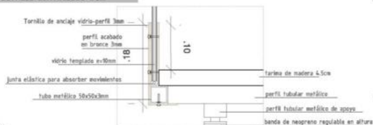
DETALLE: QUITAMIEDOS 1/5m
