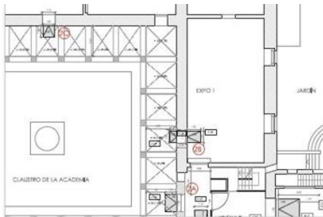
ESTADO MODIFICADO - PLANTA (1/150)
