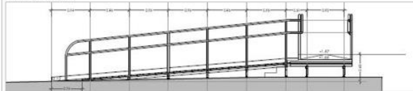
SECCIÓN LONGITUDINAL (1/40)
