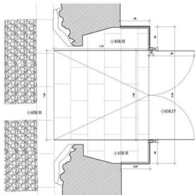
DESPIECE DE ACSITALAMIENTO e.1/50m
