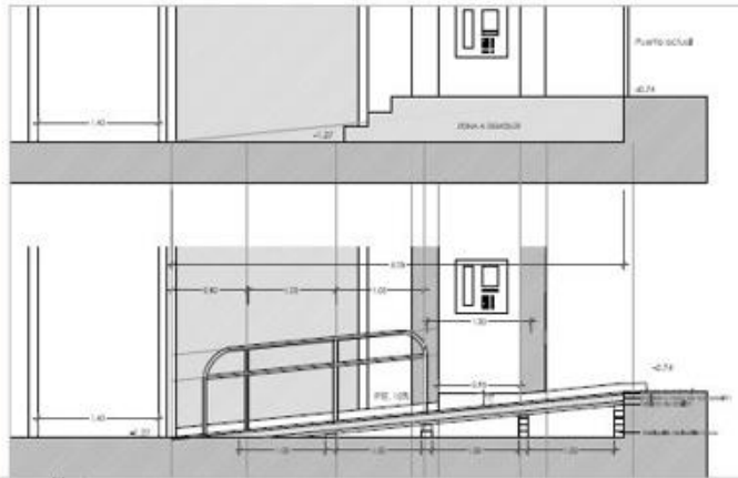
SECCIÓN LONGITUDINAL (1/40)
