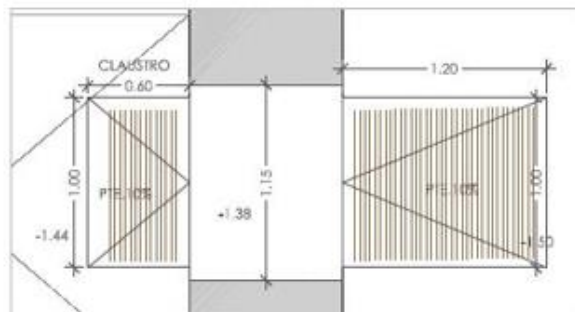
PLANTA (1/20)
