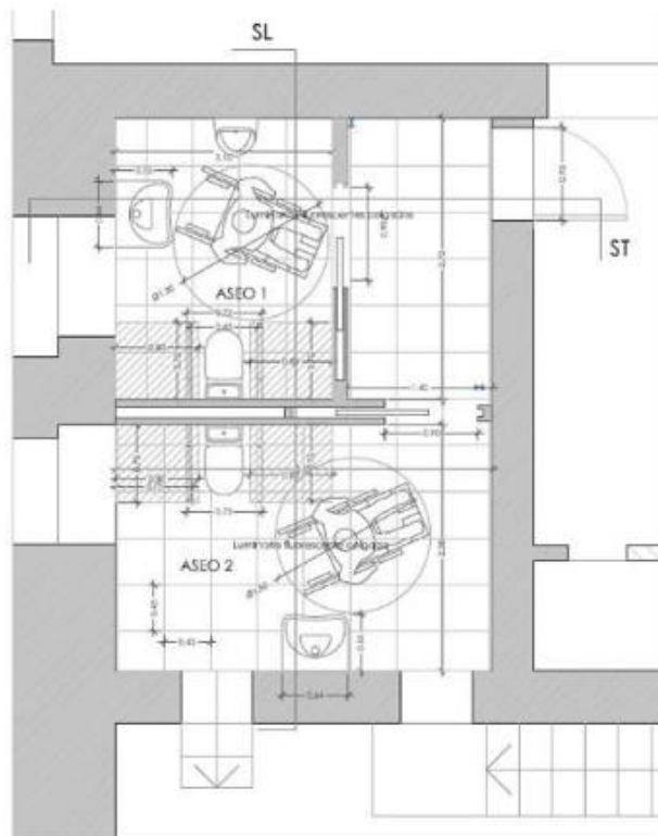
ESTADO MODIFICADO PLANTA (1/50)
