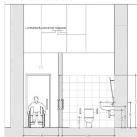
SECCIÓN LONGITUDINAL (1/40)
