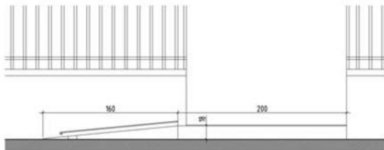
Sección longitudinal
