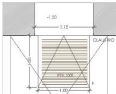
PLANTA (1/20)
