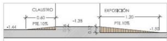
SECCIÓN (1/20)
