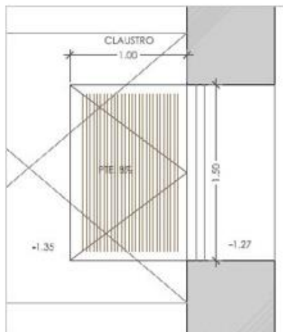
PLANTA (1/20)
