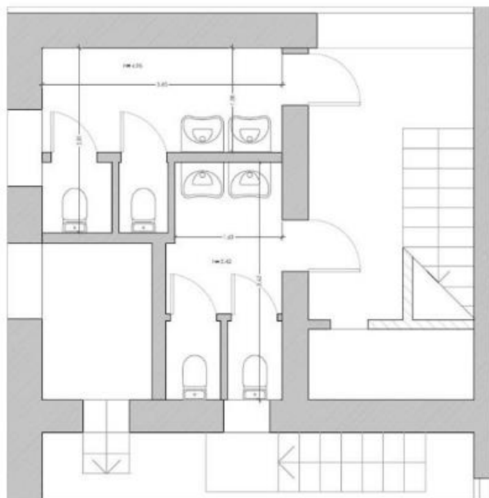
ESTADO ACTUAL -PLANTA (1/50)
