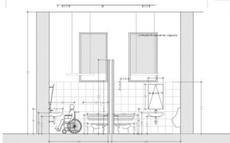
SECCIÓN TRANSVERSAL (1/40)
