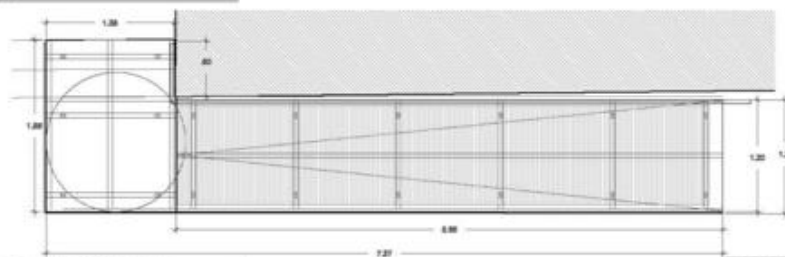
DETALLE: QUITAMIEDOS 1/5m
